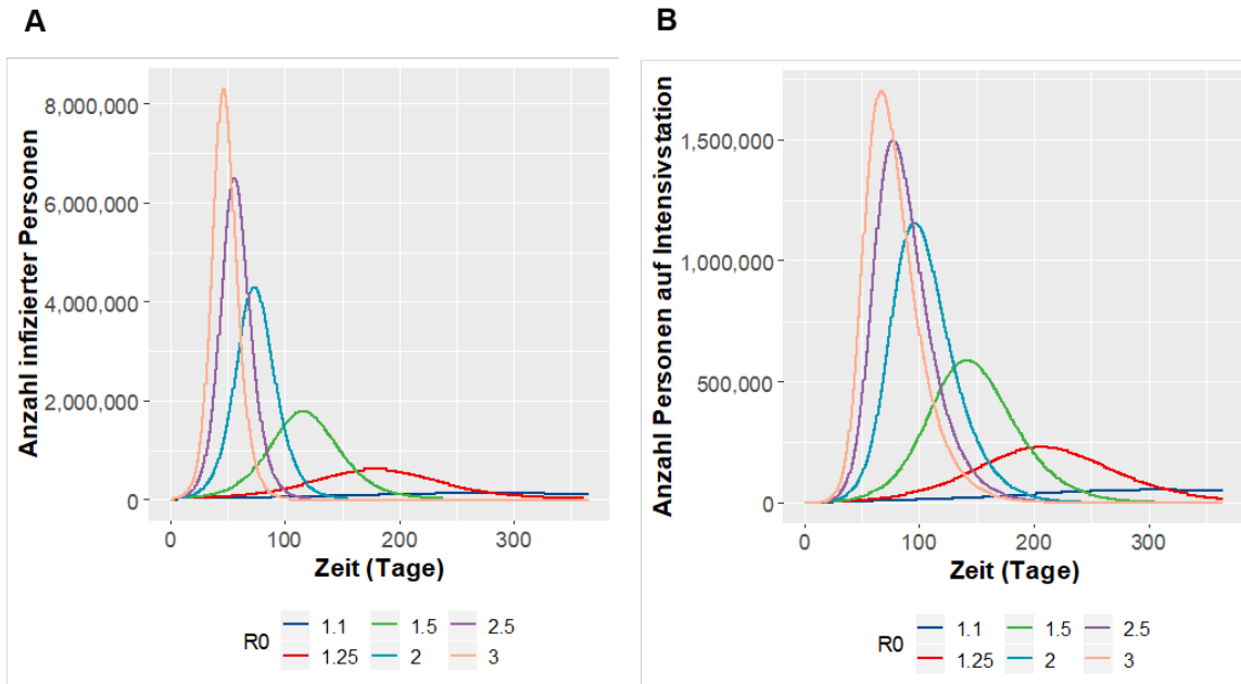
Abb. 1. Zeitlicher Verlauf der Epidemie für unterschiedliche Basisreproduktionszahlen ( R_0 )/effektive Reproduktionszahlen. Dies stellt die Auswirkungen von Kontrollmaßnahmen durch unterschiedliche Reproduktionszahlen nach Einführung der Maßnahmen auf die COVID-19 Fallzahlen dar. Auf der horizontalen Achse ist die Zeit angegeben und auf der vertikalen Achse die Anzahl an Personen, die zu einem Zeitpunkt (Panel A) infiziert sind oder (Panel B) auf einer Intensivstation behandelt werden müssen. So gibt es zum Beispiel an Tag 50 bei einer Reproduktionszahl von 2,5 5.687.270 infizierte Personen (Panel A), bei einer Reproduktionszahl von 2 würden an Tag 100 1.140.233 Personen intensivspflichtig sein
